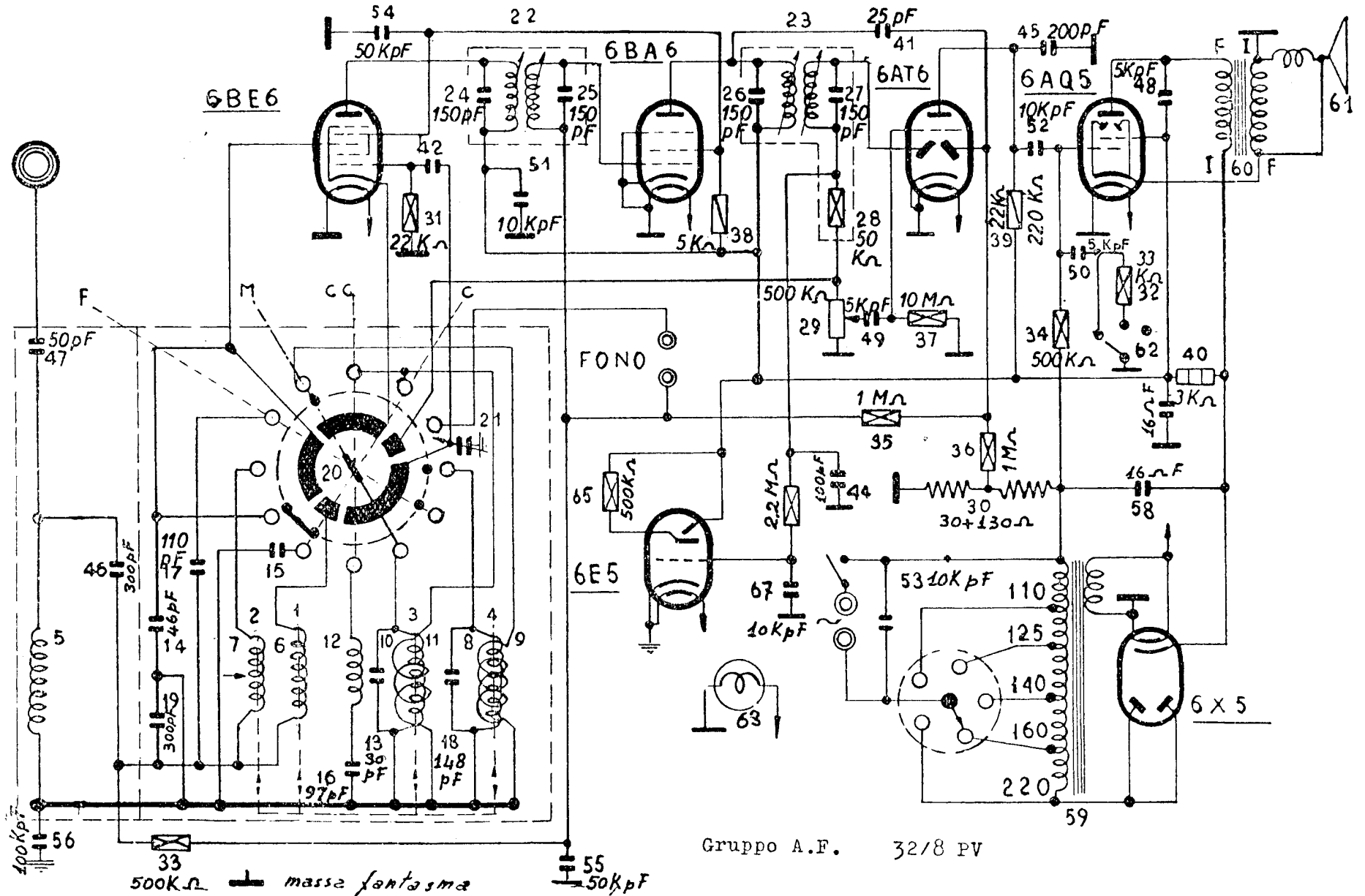
UNDA RADIO - Mod. 63/14. Supereterodina a 3 gamme d'onda: 16-29; 29-52; 184-578 m. Media frequenza 467 kc. Consumo: W 45, cc. 55 mA, ca. 290 mA. Potenza d'uscita 2 watt.
